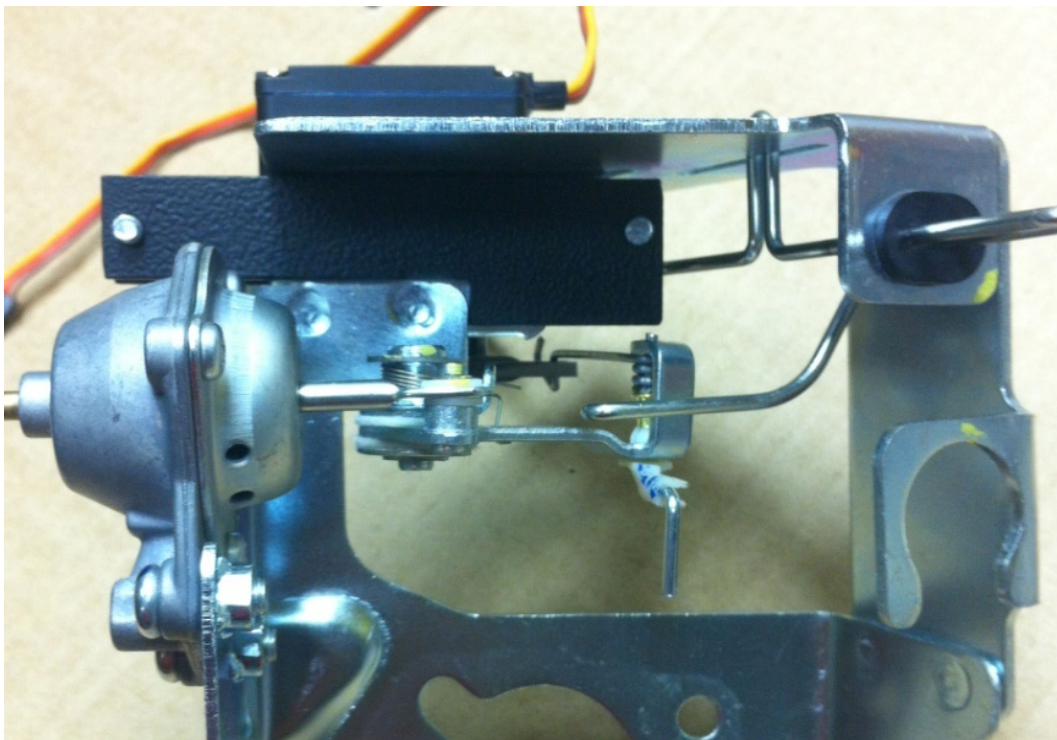
Рисунок 3 Крепление актуатора. Вид с обратной стороны
