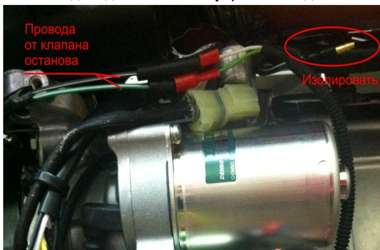
Рисунок 7 Размещение проводов топливного клапана и блока MS
