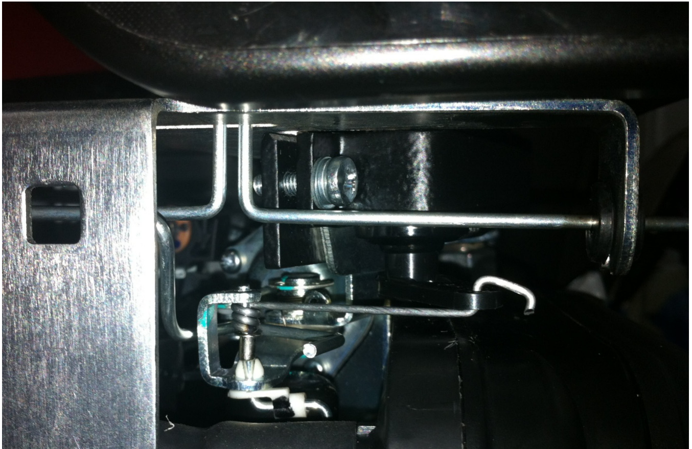
Рисунок 5 Вид актуатора на двигателе электростанции
